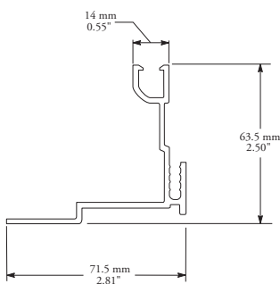
1. 40RF001564405 Matl: 6061-T6 Aluminum
