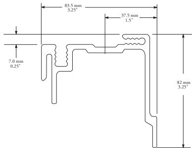
1. 39RFDF1398 Matl: PVC
