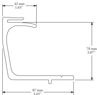
1. 40RF006455601 Matl: PVC
