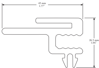
1. 39RFDF1398 Matl: PVC
